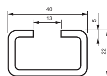
SH-E (длина 1м)
